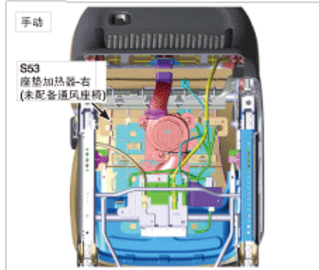
180. 助手席座椅
