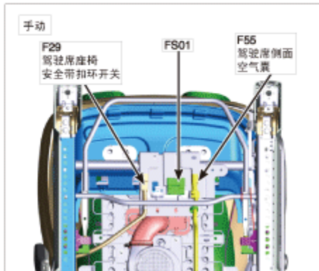
176. 驾驶席座椅
