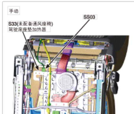
177. 驾驶席座椅
