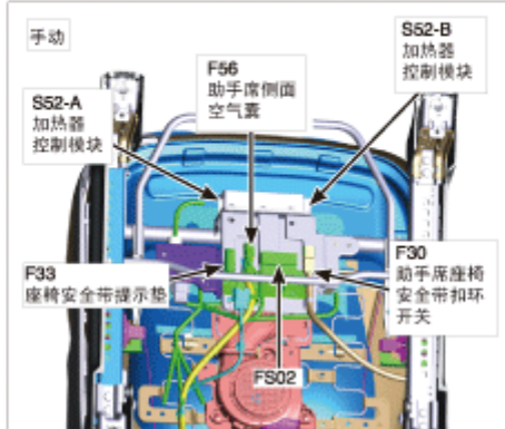
179. 助手席座椅
